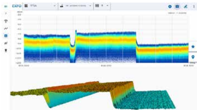
Figura 1. Espectro de persistência em tempo real com visualização 3D.
